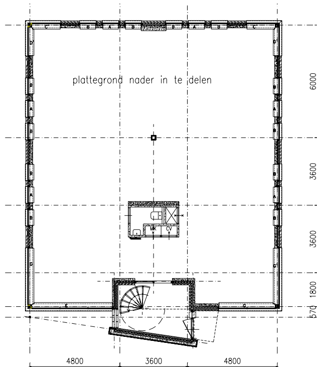
Plattegrond villa+, begane grond, gebouw 1 en 5 gesp.
