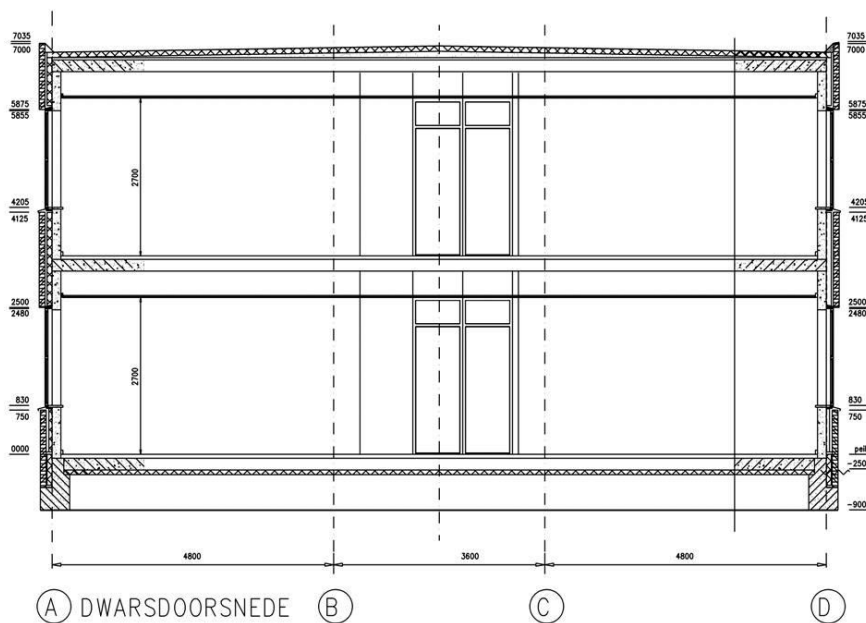
Dwarsdoorsnede villa, gebouw 1, 3 gesp., 4 en 5 gesp. voorzijde
