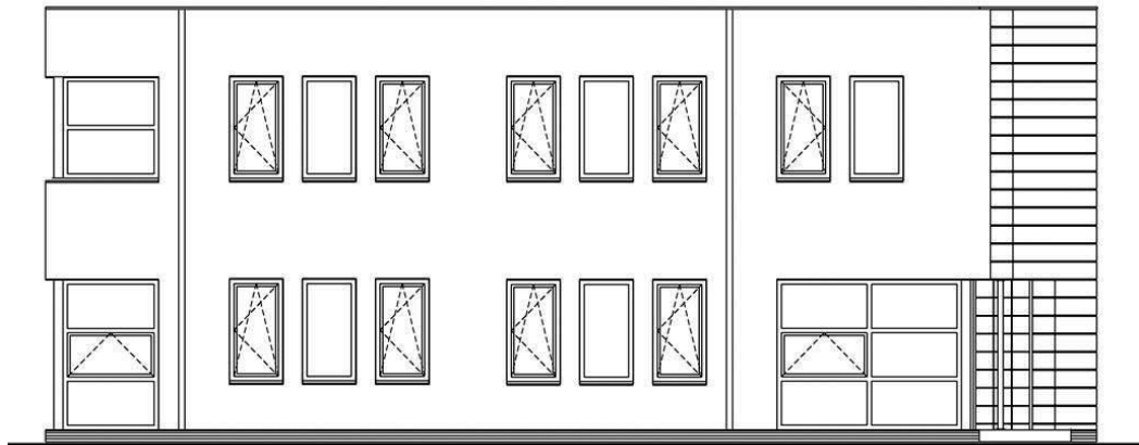
Zijgevel villa+
