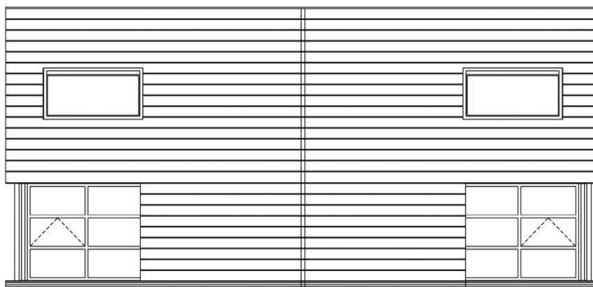
Voorgevel 2/1 kap, gebouw 2
