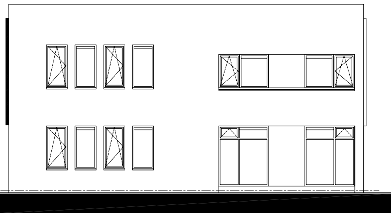
Achtergevel villa
