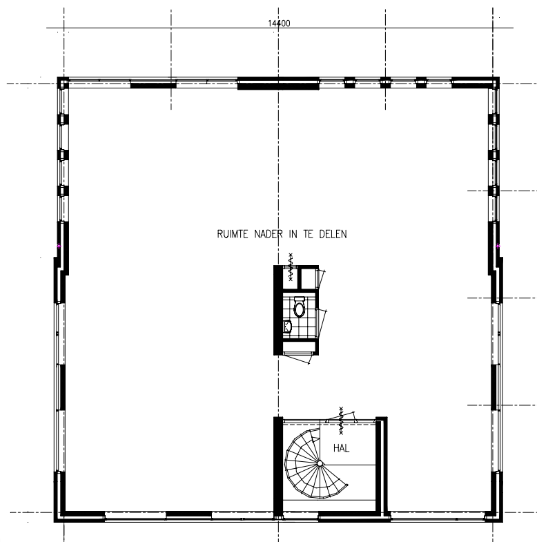
1° verdieping villa
