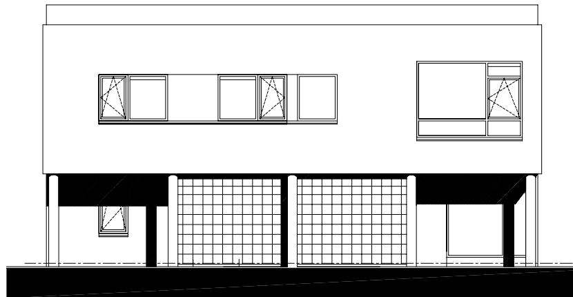
Voorgevel villa
