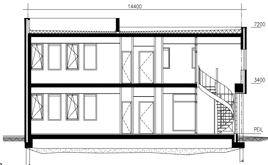
Doorsnede 2/1 kap
