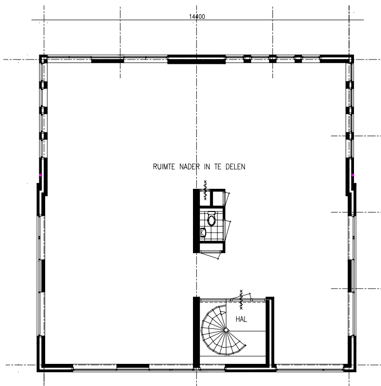
1° verdieping villa
