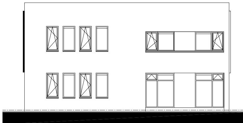
Achtergevel 2/1 kap
