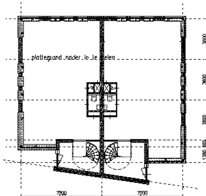
Gebouw 2, 2/1 kap, begane grond
