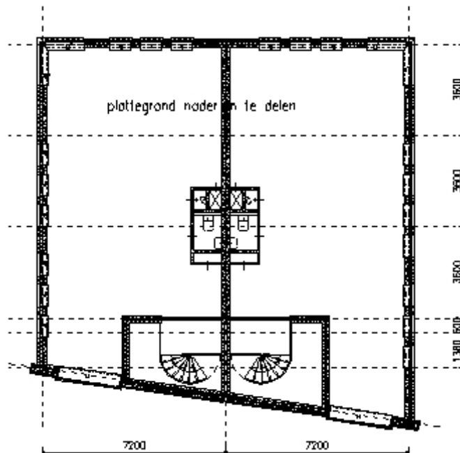
Gebouw 2, 2/1 kap, verdieping
