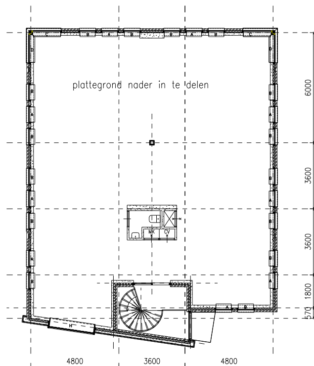
Gebouw 1, Villa, verdieping
